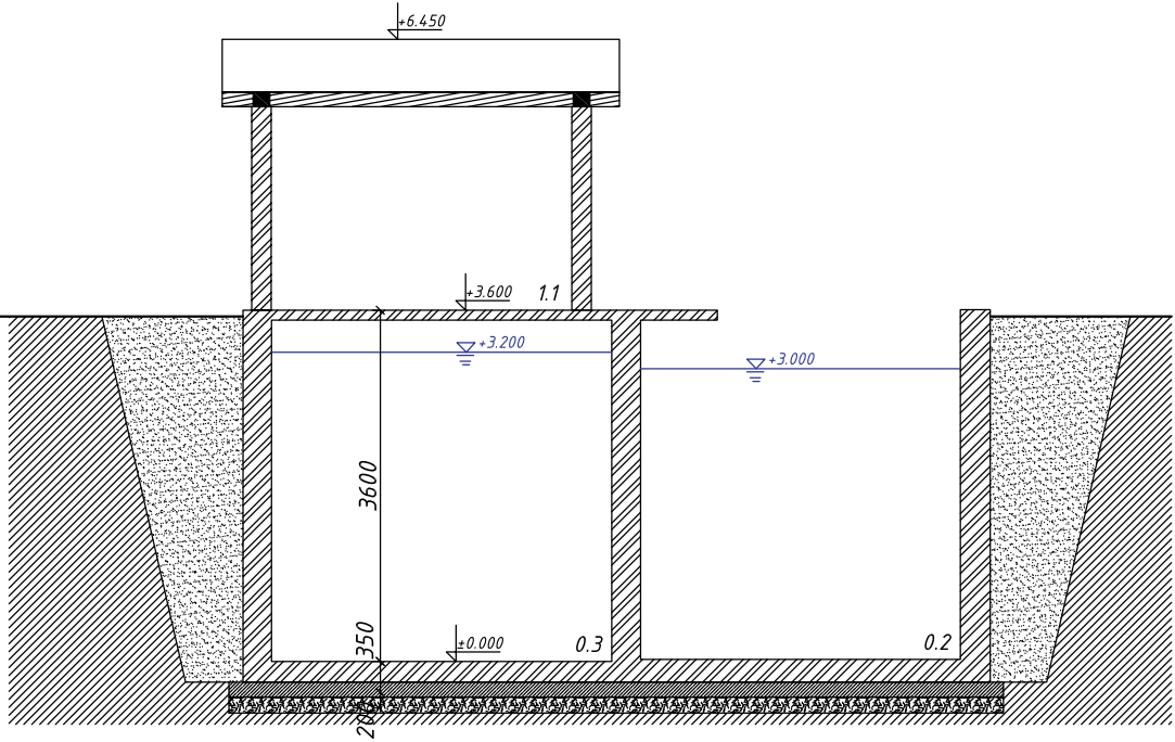
ВЕРТИКАЛЬНЫЙ РАЗРЕЗ
