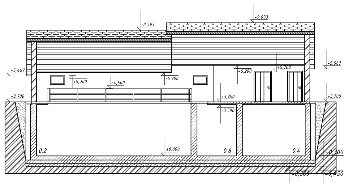
Разрез А/2
