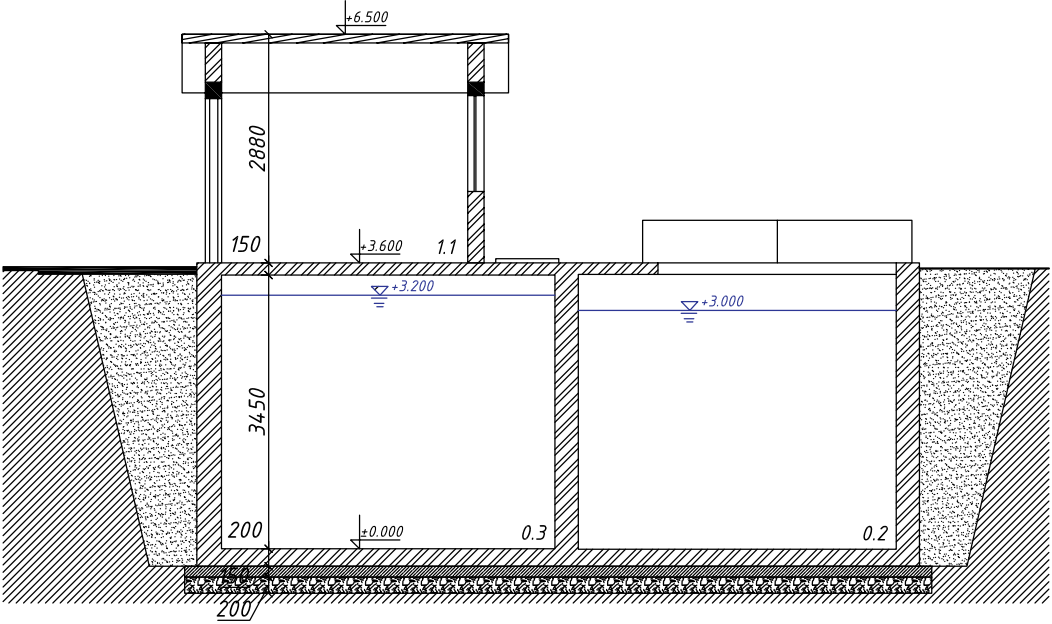
ВЕРТИКАЛЬНЫЙ РАЗРЕЗ
