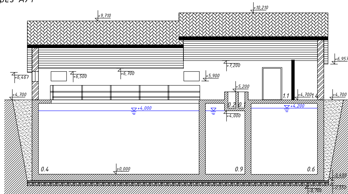
разрез A/1
