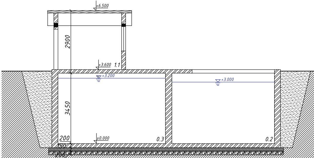
ВЕРТИКАЛЬНЫЙ РАЗРЕЗ
