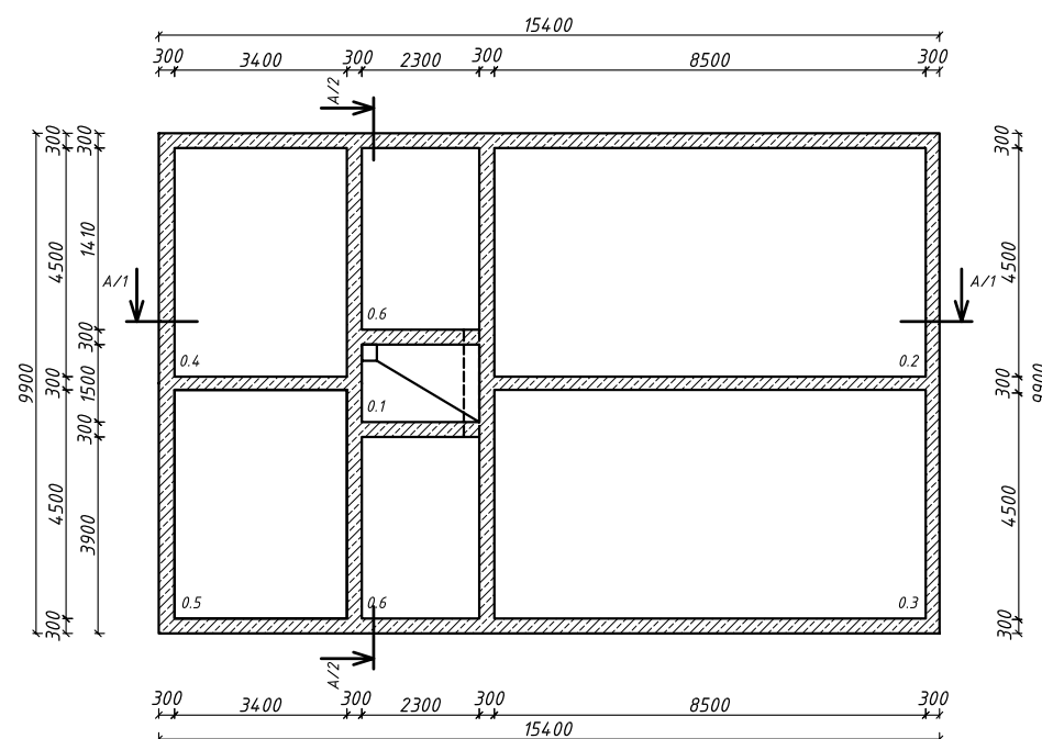
Строительные размеры:
