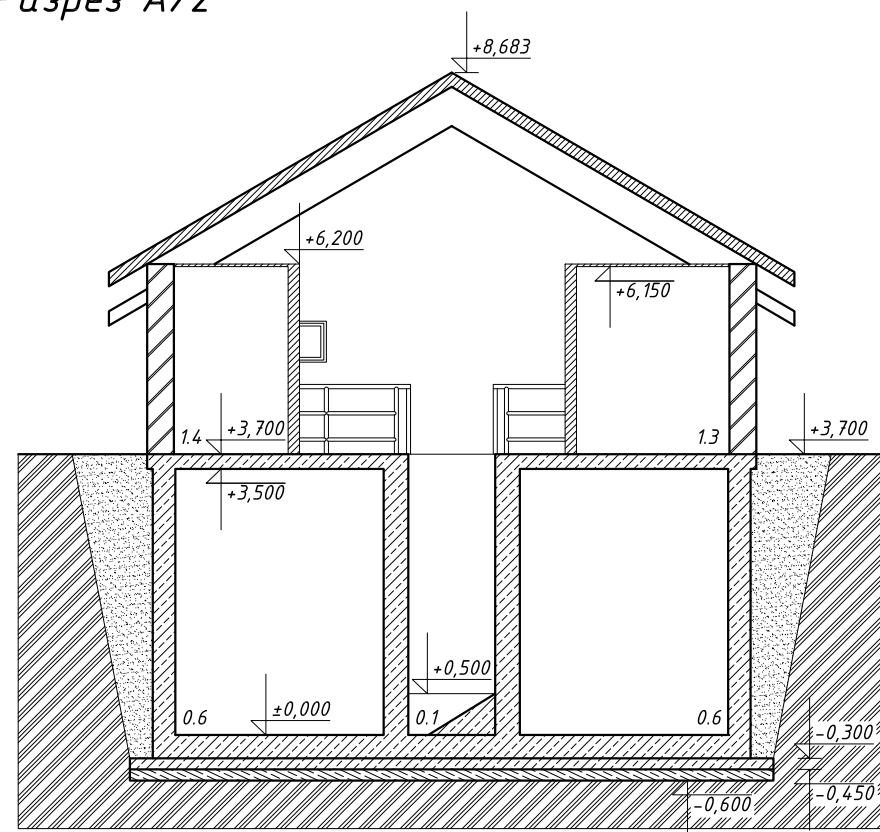
Разрез А/2
