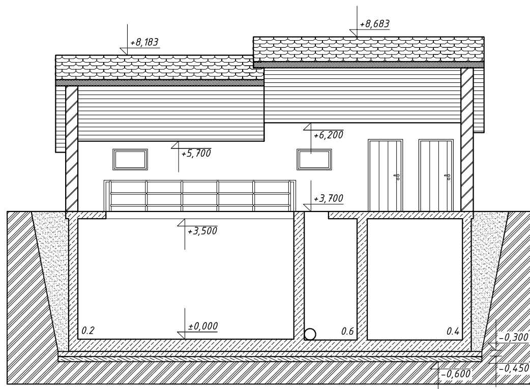
Разрез А/2
