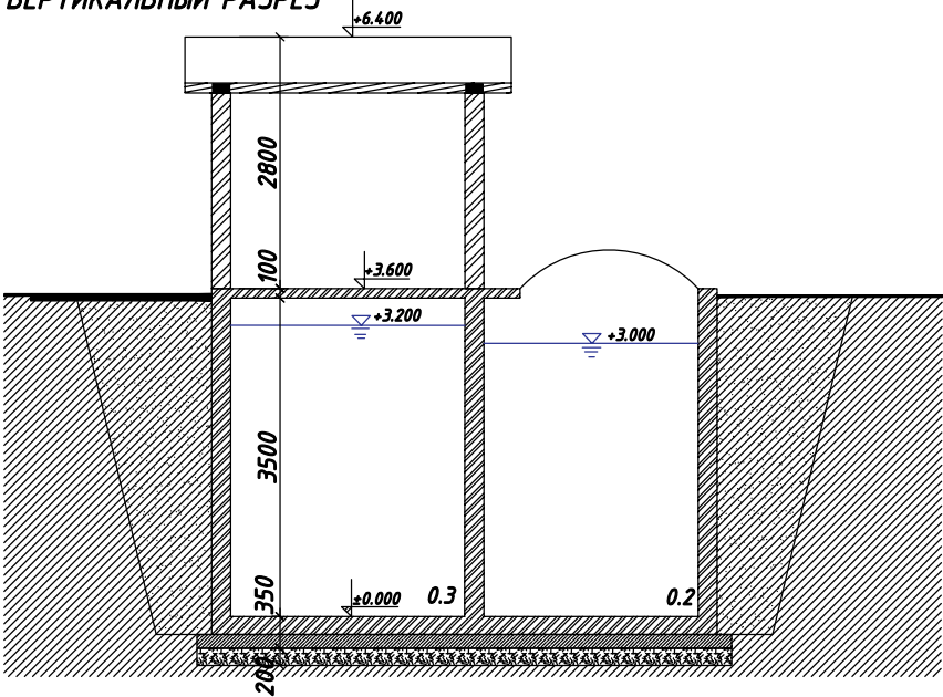
ВЕРТИКАЛЬНЫЙ РАЗРЕЗ
